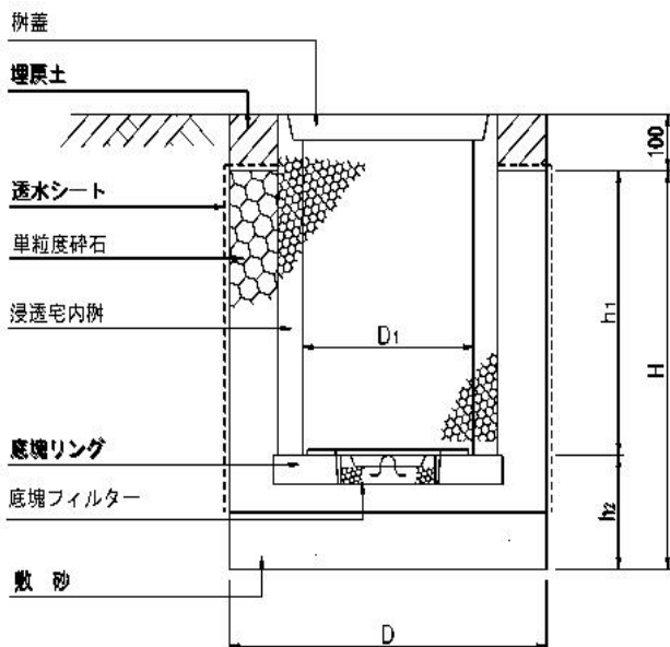
[標準構造図]EM
